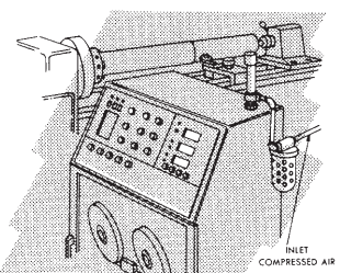
NC機械の制御盤の冷却
